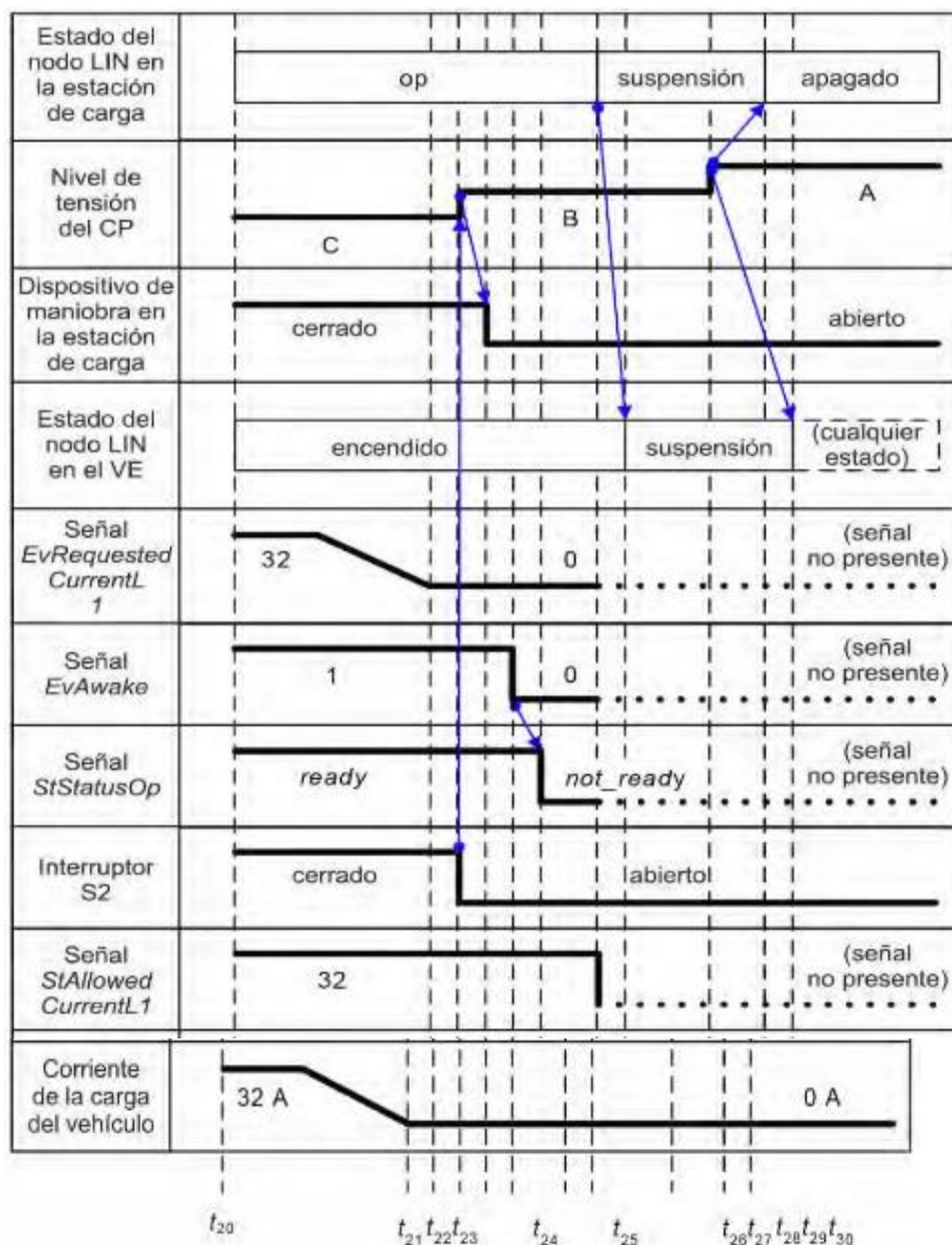
Figura D.5 Cronograma para parada normal de carga activada por el VE
