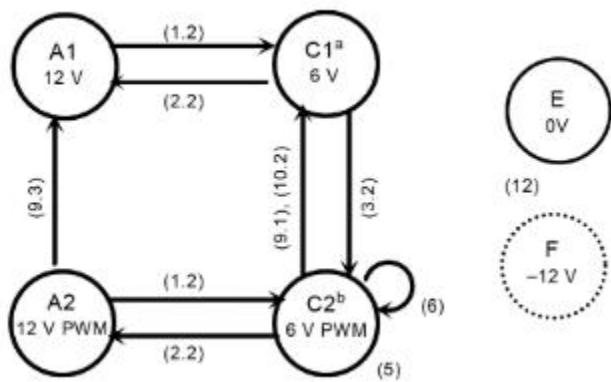
Figura A.3 Diagrama de estados para un piloto de control típico (informativo)
