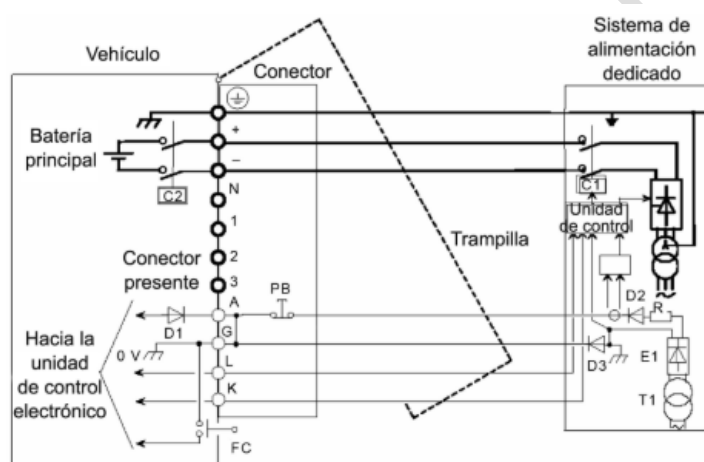
Figura C.6 Ejemplo de modo 4, caso C, utilizando el acoplamiento de vehículo universal
