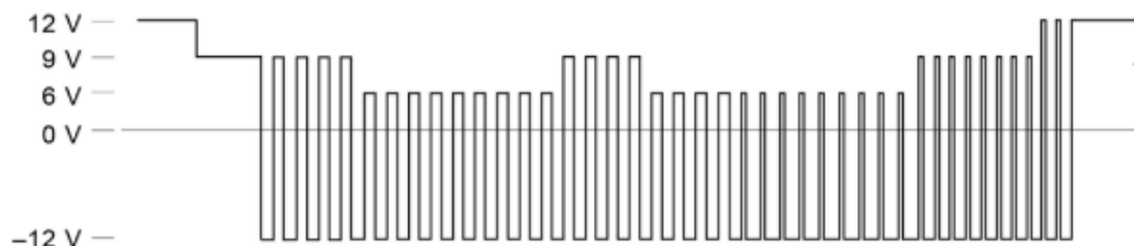
Figura A.5 Secuencia de ensayo utilizando un circuito piloto de control típico
