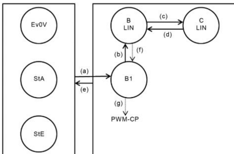
Figura D.3 Diagrama de estado del circuito piloto de control para LIN_CP (lista de leyenda en la Tabla D.5)
