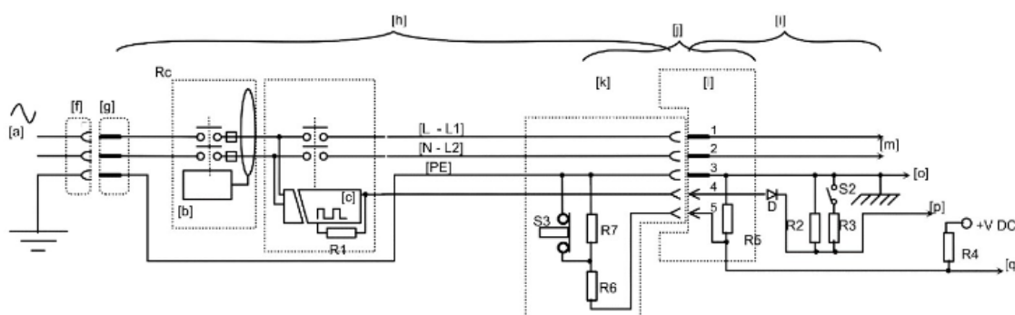
Figura C.1 Ejemplo de modo 1, caso B, utilizando circuito de proximidad como en el capítulo B.1
